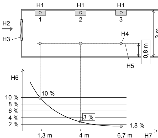
Bild 6: Berechnungsbeispiel
