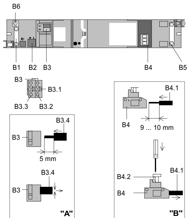
Bild 3: Anschlüsse
